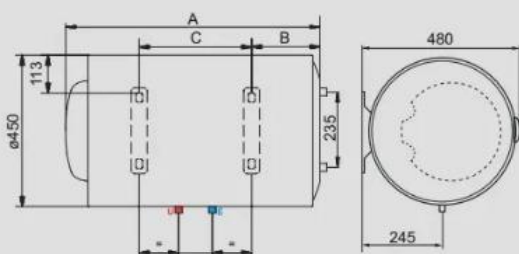
HTD (per HTS attacchi serpentino a sinistra)
