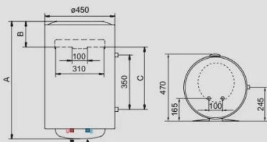
HTD (per HTS attacchi serpentino a sinistra)
